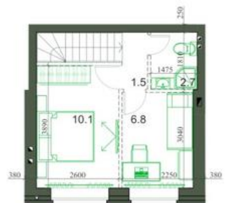
T46 2 этаж
